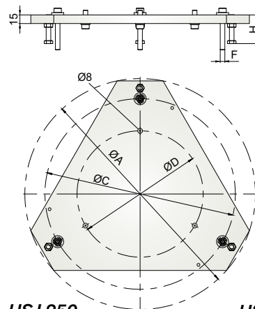
USJ 250
