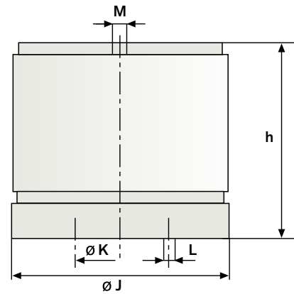
SRC-N 63-2 SRC-N 100-2
