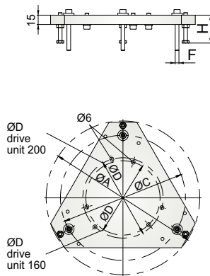
USJ 160/200
