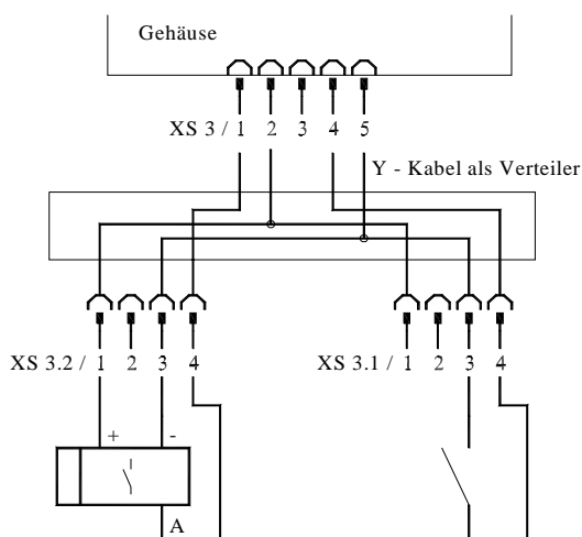
Anschluß eines Sensors und eines Kontaktes mit Adapter. Termination of a sensor and a contact by adapter.
